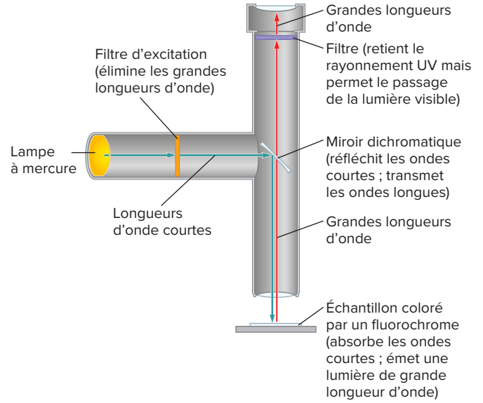
Figure 2.12 La microscopie à épifluorescence. Les principes du fonctionnement du microscope à épifluorescence.
