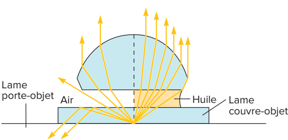
Figure 2.5 L'objectif à immersion d'huile. Objectif à immersion opérant dans l'air et dans de l'huile à immersion.
