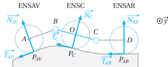
► Figure 1.41. Configuration plane du châssis en évolution sur le sol.
