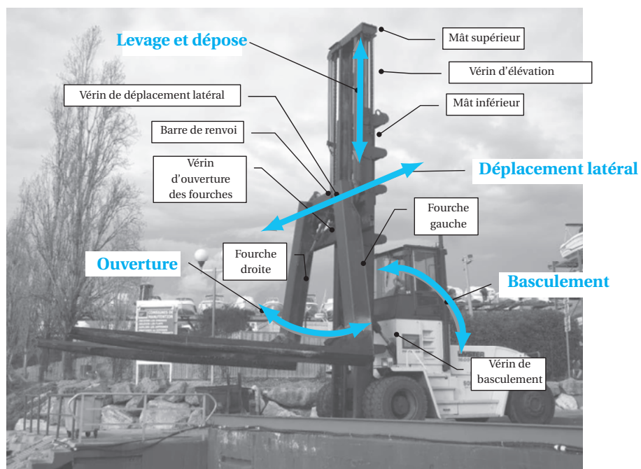
► Figure 1.36. Éléments du chariot élévateur étudié et les quatre mouvements possibles.
