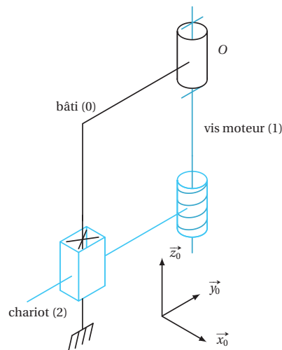
► Figure 1.11. Modèle d'un mécanisme élévateur.
