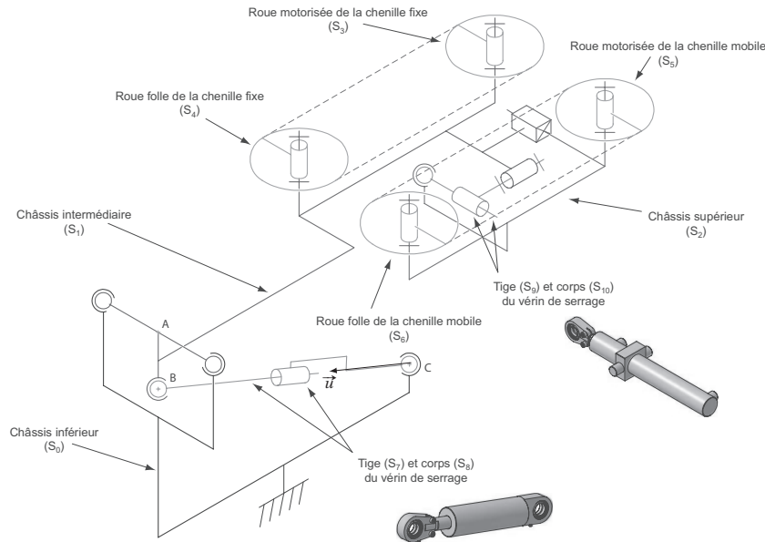
► Figure 1.34. Schéma de principe de la MTL.
