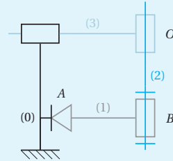
Évolution isostatique par ajout d'une pièce et d'une glissière.
