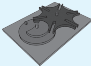
► Figure 1.43. Exemple de mécanisme de croix de Malte à 6 positions indexées.
