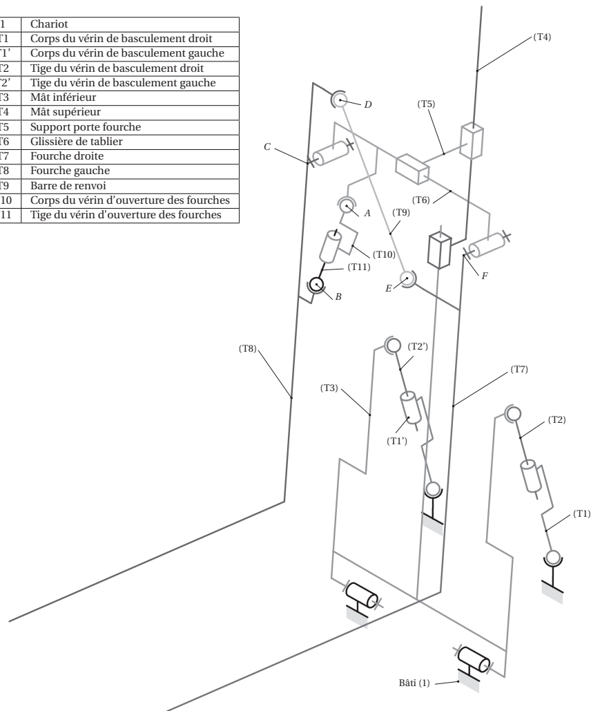
► Figure 1.37. Modèle du tablier.
