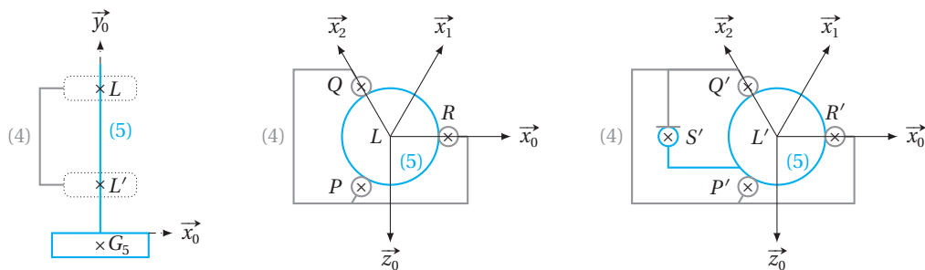
► Figure 1.32. Modélisation de la liaison entre (4) et (5).
