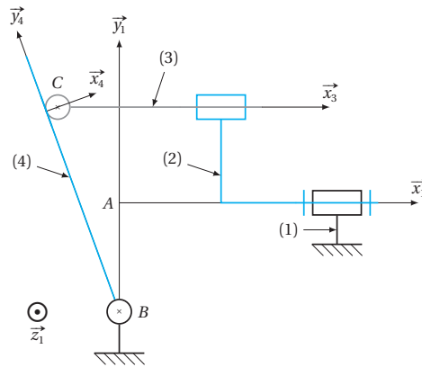
► Figure 1.10. Pompe à pistons.
