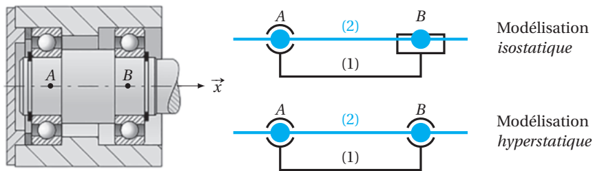
► Figure 1.1. Guidage en rotation par roulements à billes : dessin technique et modélisations isostatique et hyperstatique du guidage.
