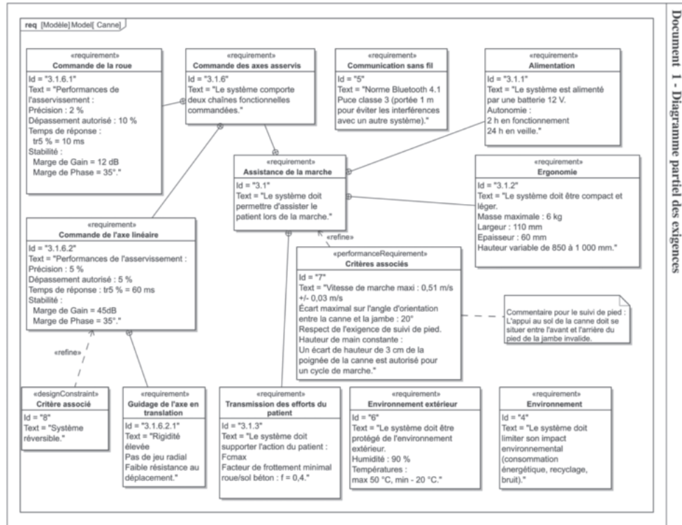
► Figure 1.17. Diagramme partiel des exigences de la canne robotisée.
