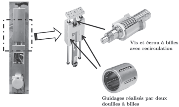
► Figure 1.18. Solutions technologiques retenues pour la transformation de mouvement et le guidage de l'axe linéaire
