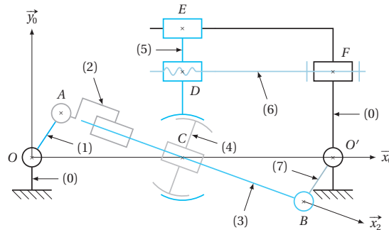
► Figure 1.15. Variateur de vitesse mécanique.
