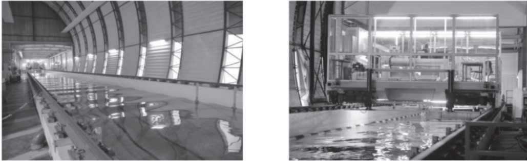
► Figure 1.30. Bassin de traction à gauche et chariot de traction à droite.
