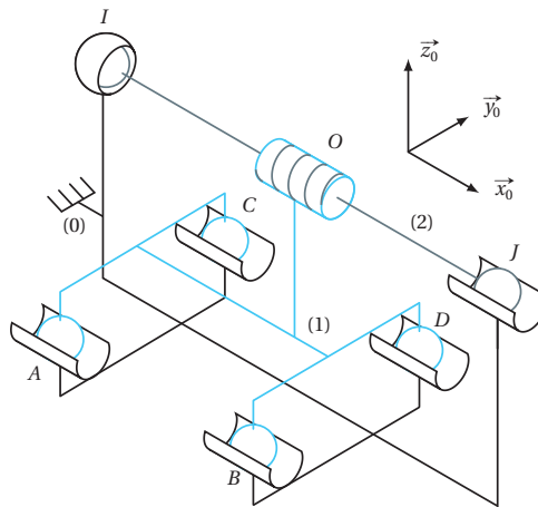
► Figure 1.14. Modèle d'une table de translation.
