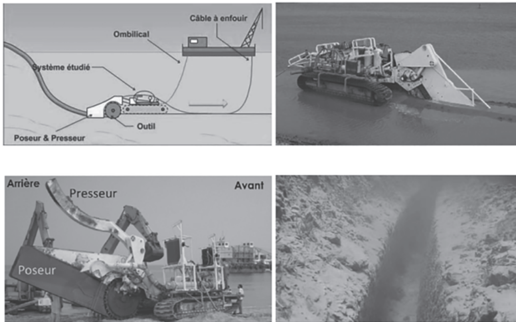
► Figure 1.33. Description du système d'enfouissement.
