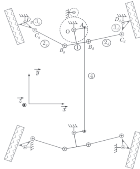
► Figure 1.28. Principe du système de direction.
