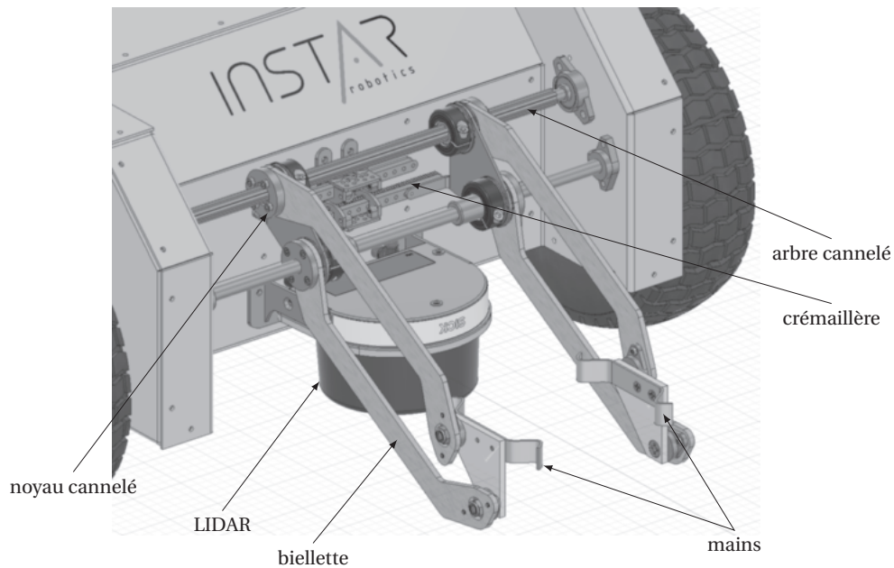
► Figure 1.22. Description du mouvement bras.
