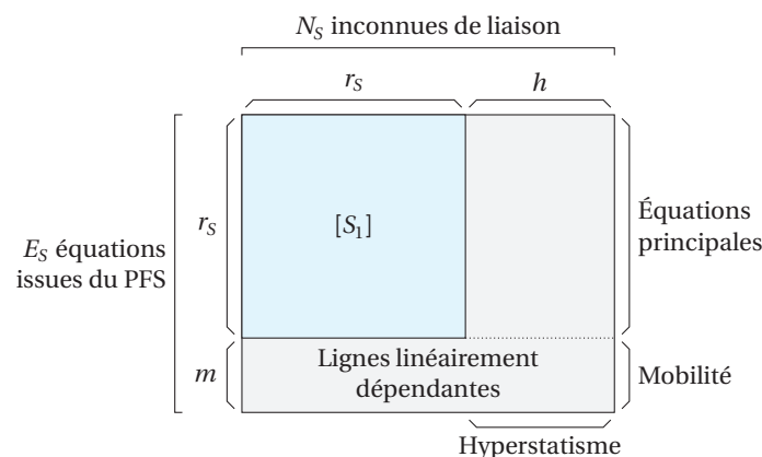
► Figure 1.7. Identification de la mobilité m et de l'hyperstatisme h d'une modélisation à partir de l'analyse de la structure de la matrice [S] issue de l'étude statique.
