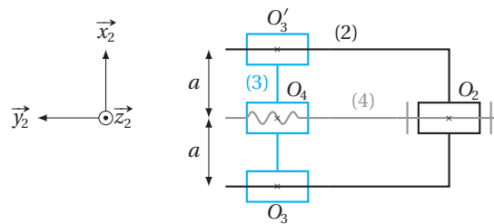
► Figure 1.19. Modèle cinématique de la transformation de mouvement et du guidage de l'axe linéaire.
