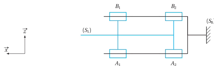
► Figure 1.24. Modélisation simplifiée des liaisons entre la crémaillère et le châssis.
