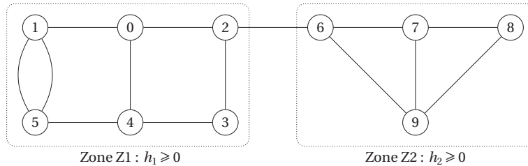
► Figure 1.4. Structure dite « hybride » de degré d'hyperstatisme h = h_1 + h_2 .
