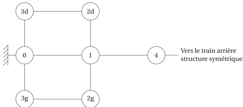
► Figure 1.29. Graphe des liaisons du train avant de la direction.
