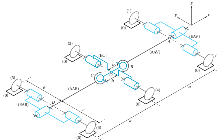
► Figure 1.40. Schéma cinématique de la plateforme.
