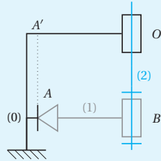
Solution initiale, contrainte en distance \|\vec{AB}\| = \|\vec{A'O}\| .
