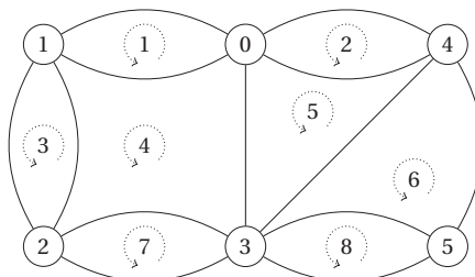
► Figure 1.5. Graphe des liaisons de nombre cyclomatique \gamma = N_L - N_p + 1 = 13 - 6 + 1 = 8 , soit 8 boucles indépendantes (par exemple celles indiquées sur la figure).
