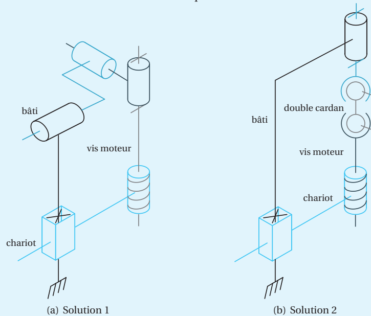
► Figure 1.42. Modèle d'un mécanisme élévateur modification.
