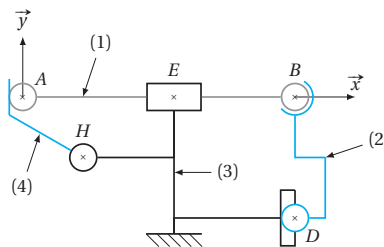
► Figure 1.9. Mécanisme de serrage.
