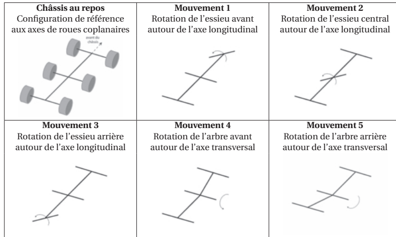
► Figure 1.39. Illustration des mouvements de déformation du châssis.
