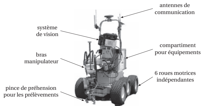
► Figure 1.38. Représentation du système ROBOVOLC.
