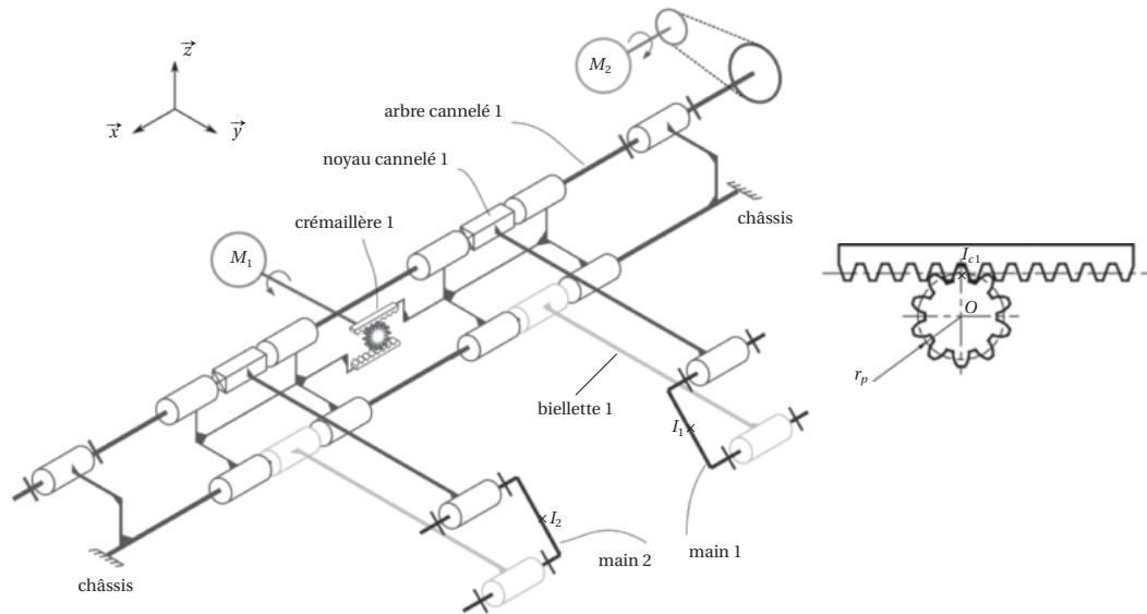
► Figure 1.23. Cinématique du système de prise des pots.
