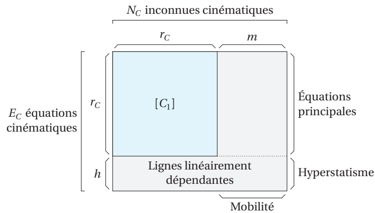
► Figure 1.6. Identification de la mobilité m et de l'hyperstatisme h d'un modèle à partir de l'analyse de la structure de la matrice [C] issue de l'étude cinématique.
