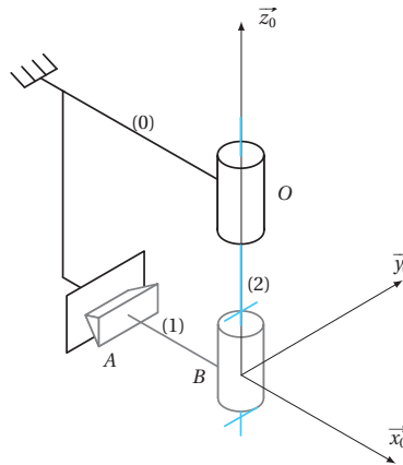
► Figure 1.12. Modèle d'une machine de traction-torsion.
