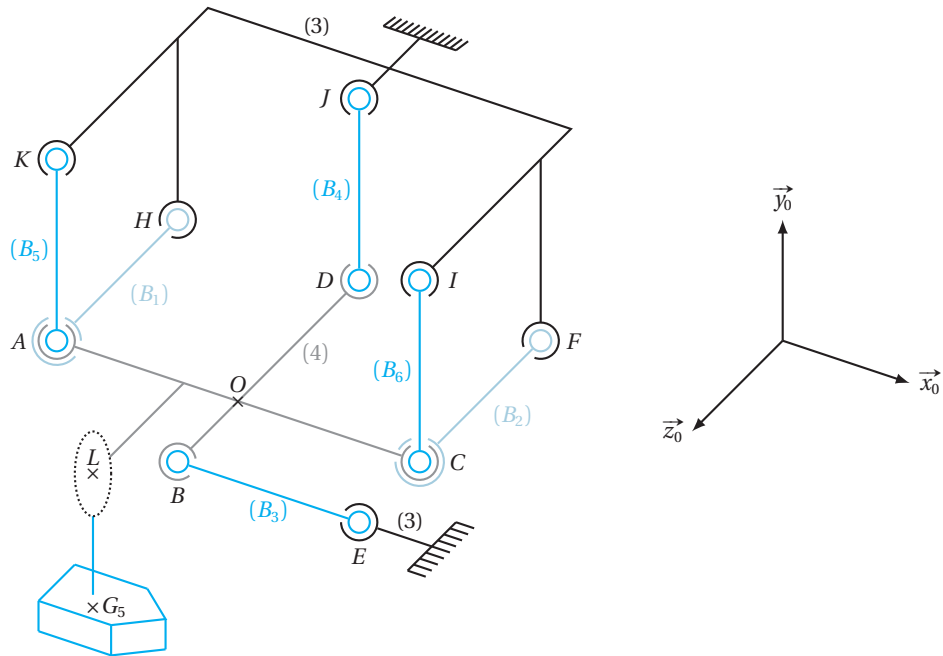
► Figure 1.31. Schéma cinématique 3D du dispositif de mesure.
